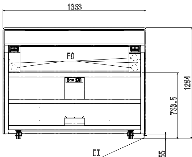
Zij aanzicht
