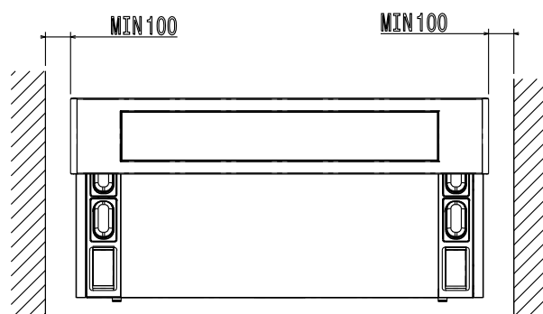
Boven aanzicht
